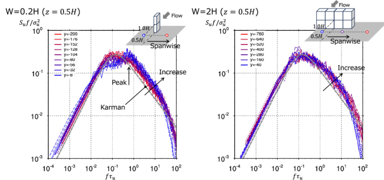
図 4. 二種類の異なる建物後流における風速のパワースペクトル密度．図中の w は模型の幅， H は模型高さ ( =0.2\text{m} )， z, y は計測位置を意味する． y=0 は模型スパン方向中心．横軸の周波数は積分時間スケールで無次元化されている．
