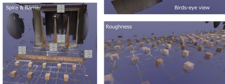
図 5. 3D スキャナーにより取得した風洞全体図と乱流生成装置の配置図. Point cloud データとして、各点には位置情報とテクスチャ（色）情報が含まれている．可視化のため、ポイントデータを拡大してラフネス等の配置を示している．
