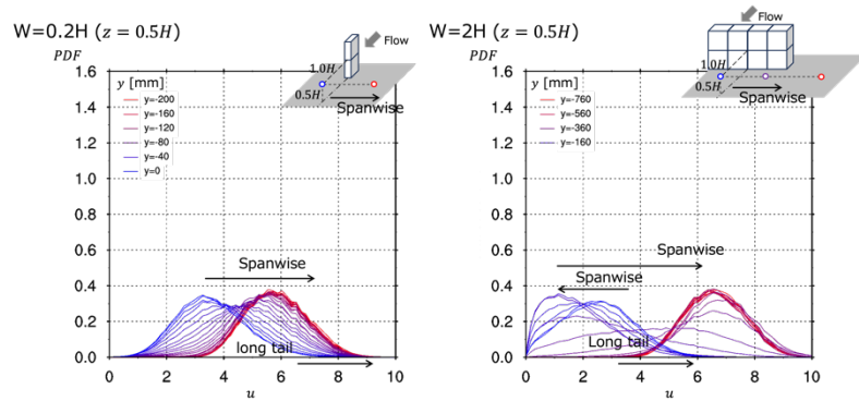
図 3. 二種類の異なる建物後流における風速の確率密度関数．図中の w は模型の幅， H は模型高さ ( =0.2\text{m} )， z, y は計測位置を意味する． y=0 は模型スパン方向中心．
