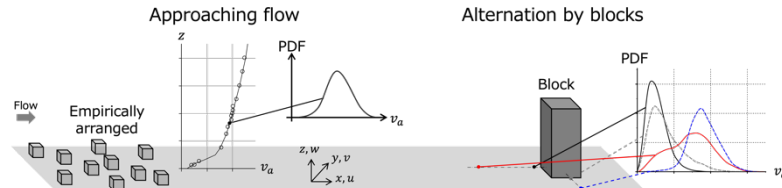
図 1. 研究対象の模式図。接近流の乱れ性状を確率分布として分析した上で、建物が生成する乱れによる確率性状の変化を分析する。
